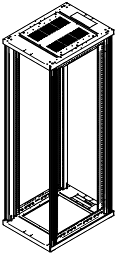
F/D800
